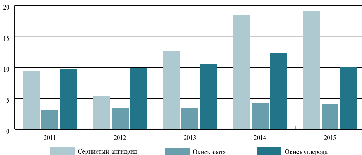
График 11.5: Выбросы загрязняющих атмосферу веществ, отходящих от стационарных источников, по ингредиентам
