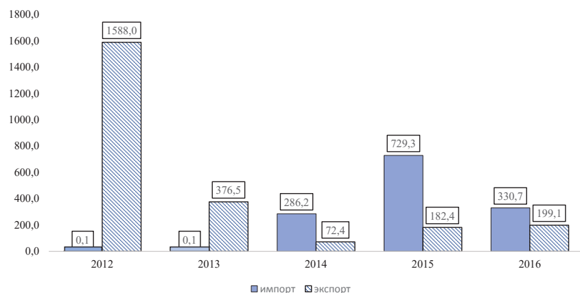
График Г3. Объем экспорта и импорта электроэнергии (млн.кВт.ч)
