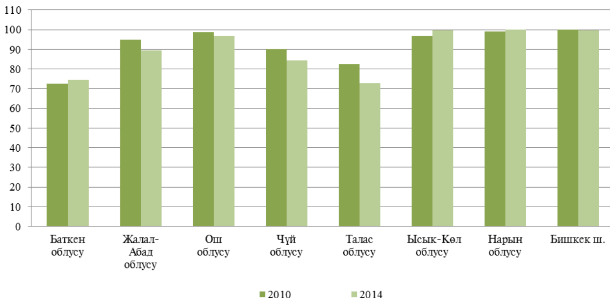
Ичүүчү сууну алууга мүмкүндүгү бар калктын аймактар боюнча үлүшү 1 (пайыз менен)
