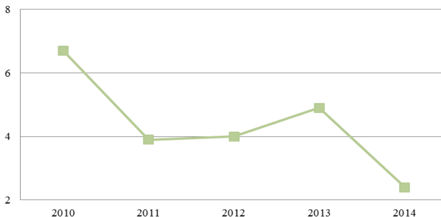
Жер бетиндеги суу объекттерине булганган агын суулардын түшүшү
