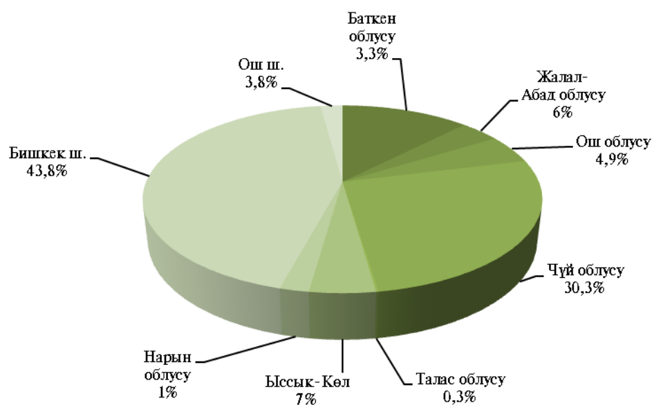
2014-жылдагы стационардык булактардан чыккан атмосфераны булгоочу заттардын аймактар боюнча таштоолору (жыйынтыкка карата пайыз менен)
